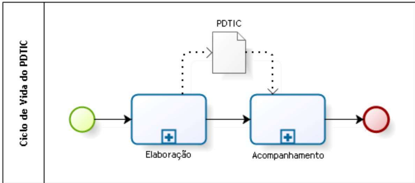
Figura 4: Macroprocesso de PDTIC
