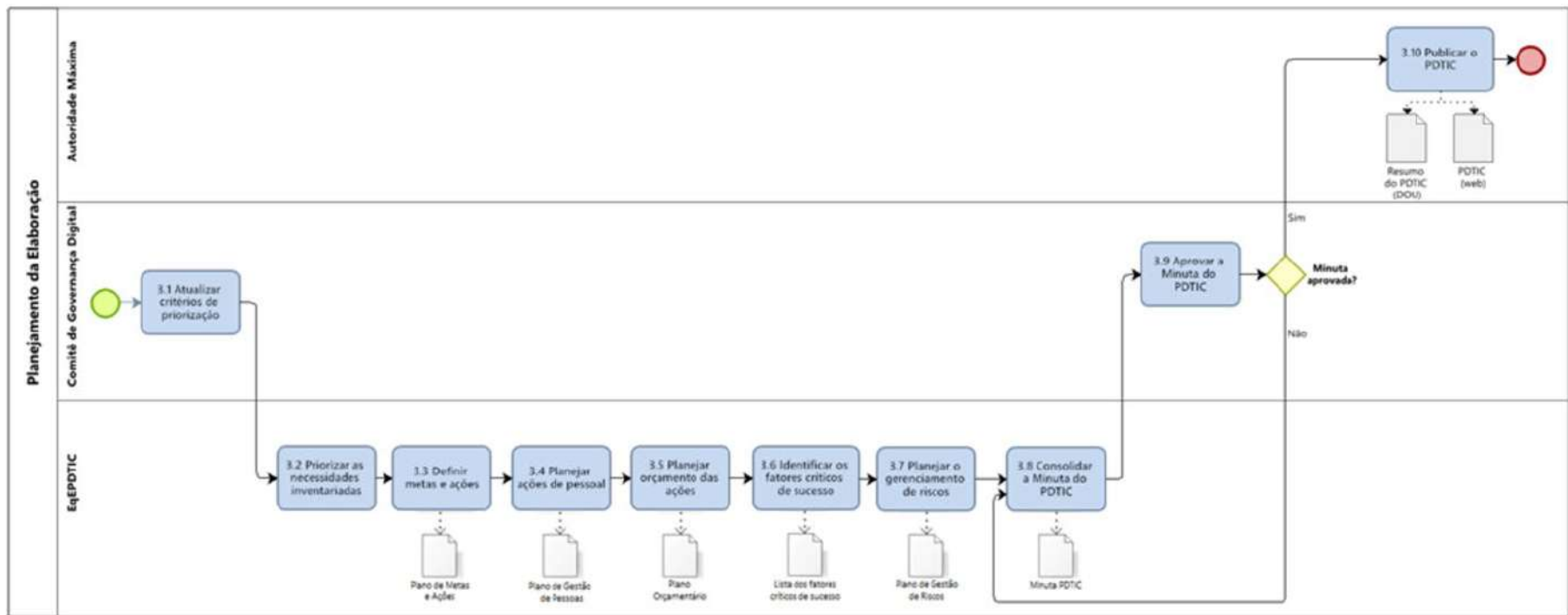
Figura 14: Subprocesso de Planejamento [Elaboração]
